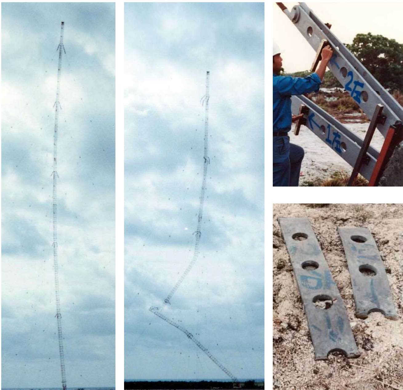
リンクプレートを切断し、倒壊させた工事例（写真はマーカス島電波塔爆破解体工事）
